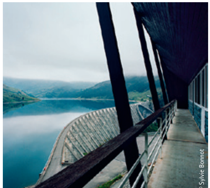
Barrage de Roselend, complexe de Roselend La Bâthie
